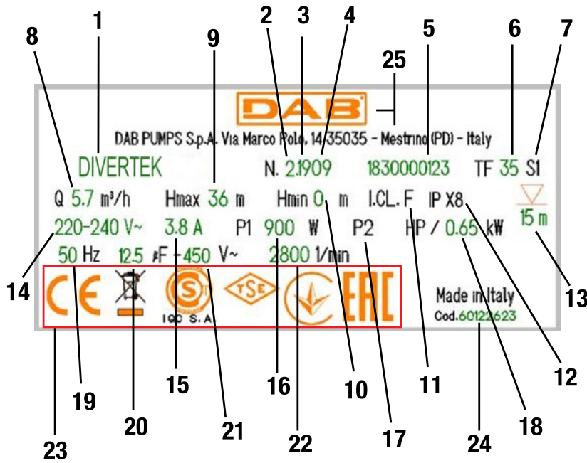
Şekil 4 Metal etiket
