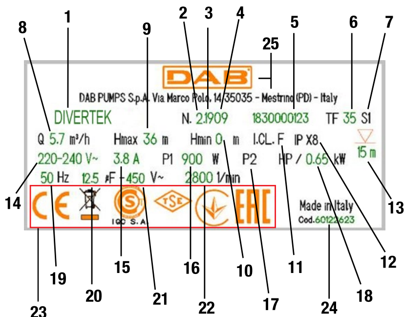
Rys. 4 Tabliczka znamionowa
